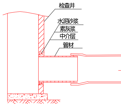
图 7.0.2 管道与检查井的连接(一)
