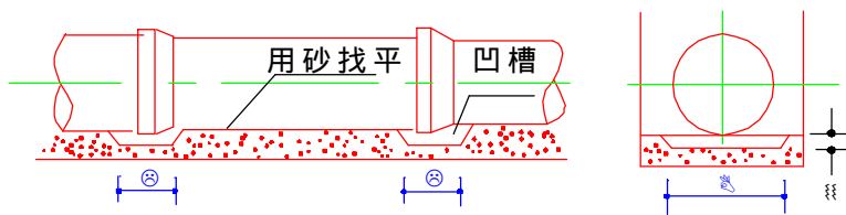
图 6.3.4 管道接口处的凹槽
