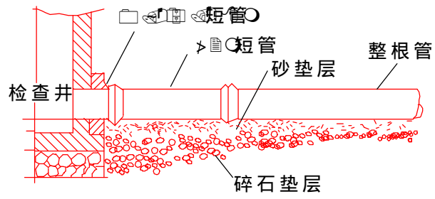
图 7.0.5 软土地基上管道与检查井连接
