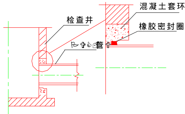
图 7.0.3 管道与检查井的连接(二)
