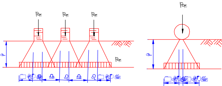
a) 顺轮胎着地宽度方向的分布 b) 顺轮胎着地长度方向的分布
