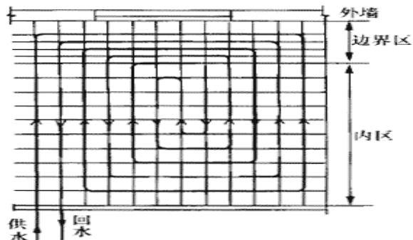
图 6 带有边界和内部地带的回折型布置
