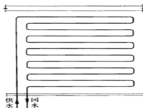
图 4 平行型布置
