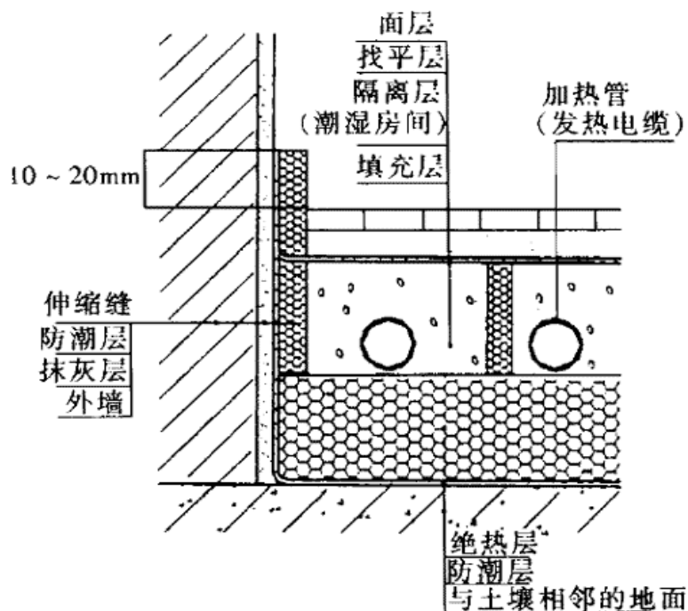
图2 与土壤相邻的地面构造示意图
