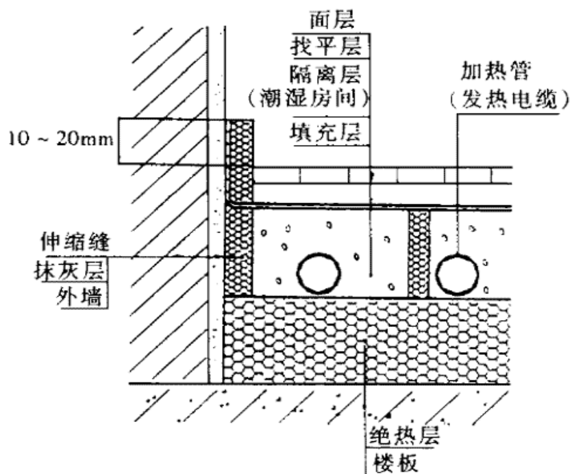
图1 楼层地面构造示意图
