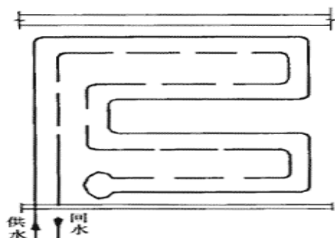
图 5 双平行型布置
