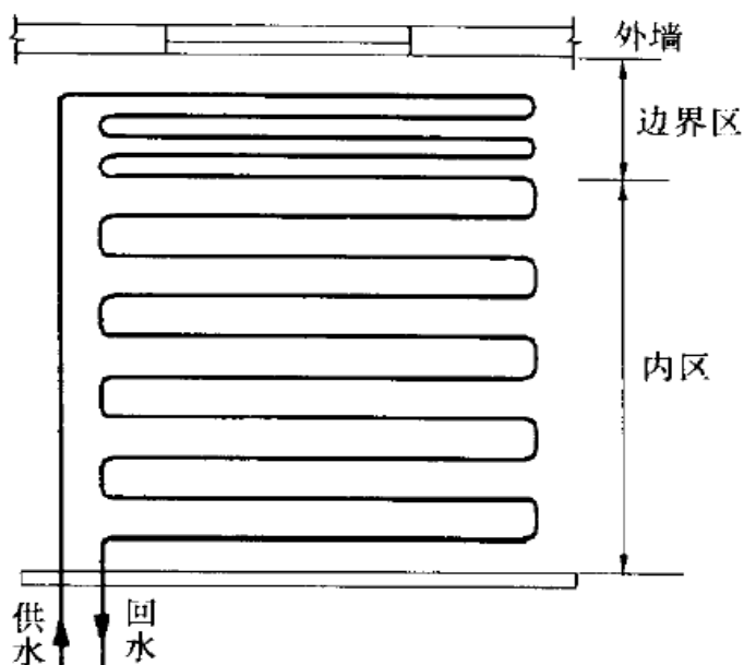
图 7 带有边界和内部地带的平行型布置
