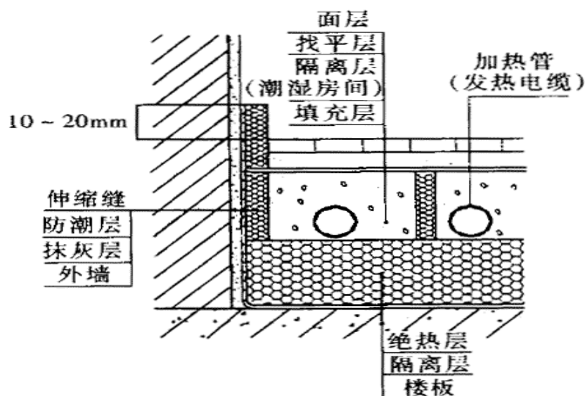
图9 卫生间地面构造示意图
